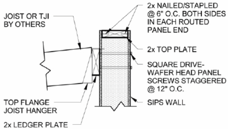
1 LEDGER DETAIL D29 1" = 1'-0"
